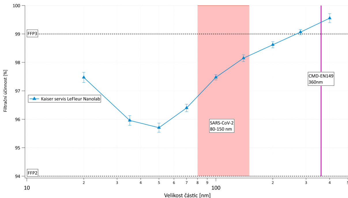
Obr.2 Velikostně rozlišená filtrační účinnost materiálu roušky LeFleur s Nanolab aktivním filtrem pro čelní rychlost 10,6 cm/s.
